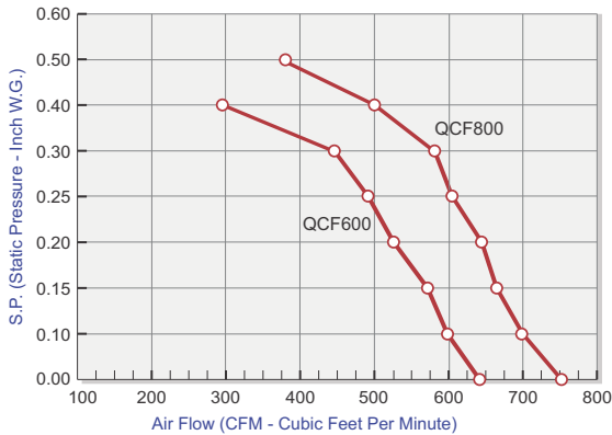
QCF600, QCF800 FAN DATA
